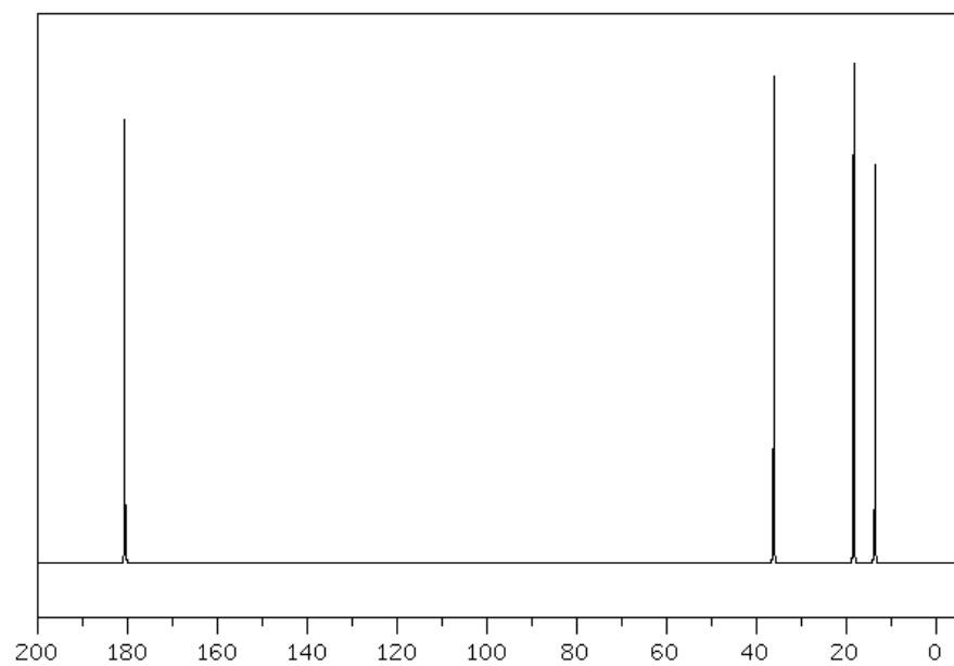
A: Butanoic acid
